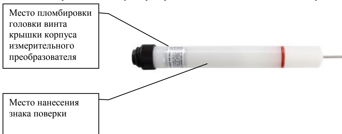
Рисунок 7 - Внешний вид, место нанесения знака поверки и пломбирования от несанкционированного доступа преобразователя влажности Rotronic модификации HC2-S3C03
